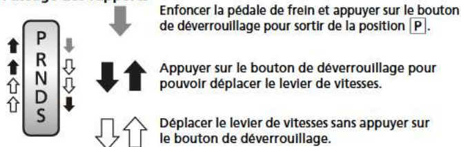
Levier de vitesses
